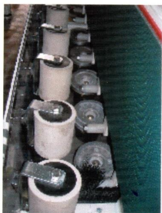
Cabeças Planas e Rolos de Pressão
